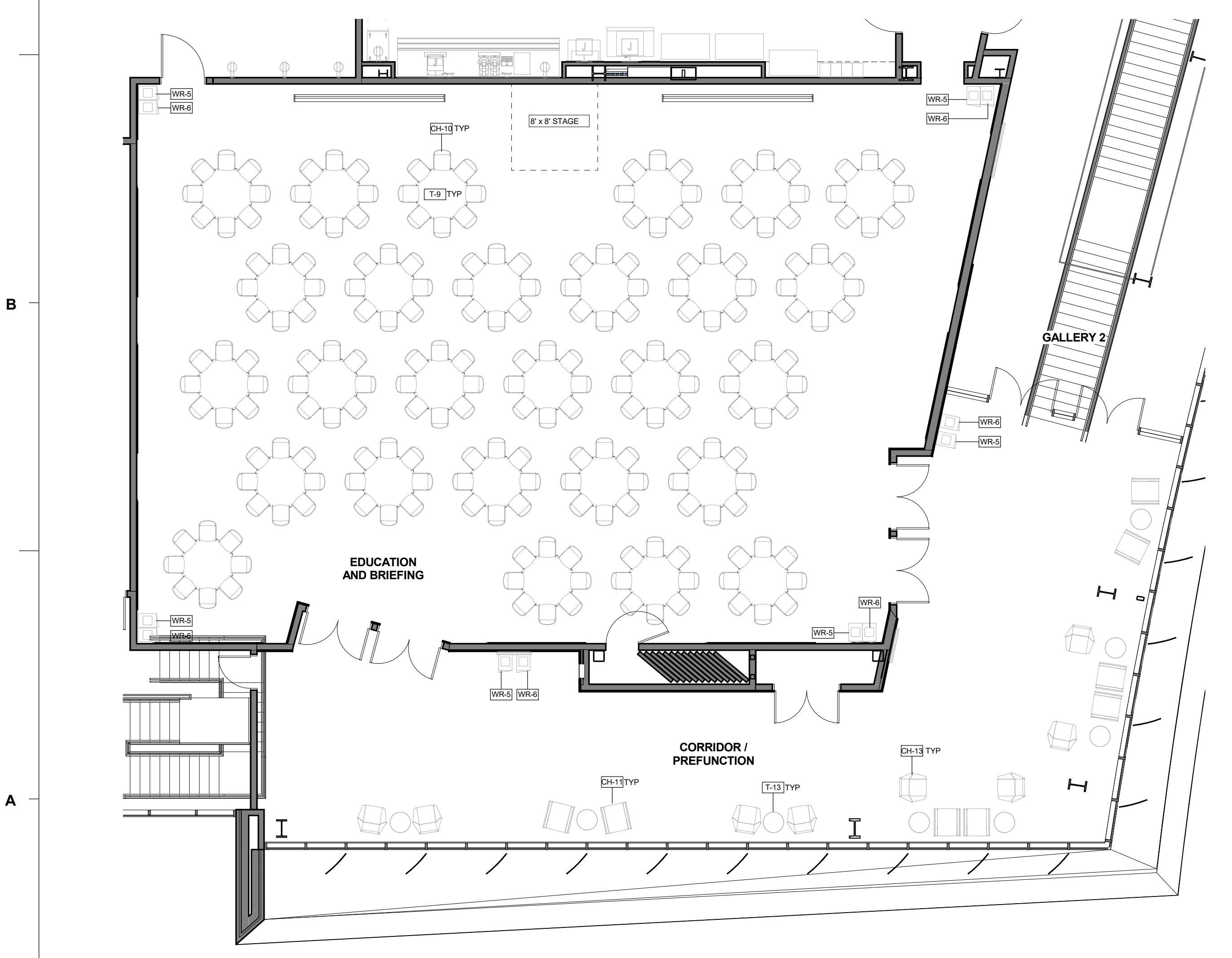
A1 BANQUET SET UP 1/8" = 1'-0"
